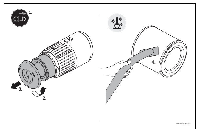
fig. 10 Heqja dhe pastrimi i filtrit
